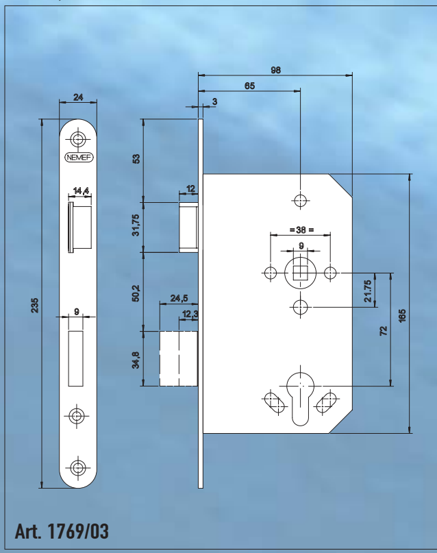
Fh-Einsteckschlösser für Feuerschutzabschlüsse bis T 120 nach DIN 18250 (Teil 1) und zertifiziert nach EN 179, Rechts und Links verschieden
