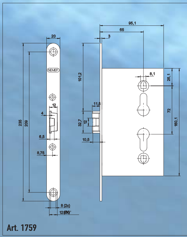
Spezial-Einsteckschloß, Rechts und Links verwendbar
